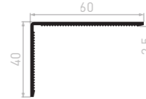
CE2530C Cornière 60X40X2,5 Crantée 10 barres de 6 ml / paquet 600 barres de 6 ml / container
