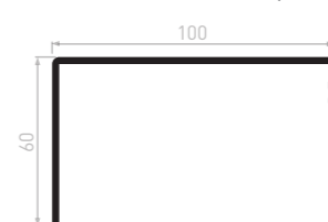
CE2521 Cornière 100X60X2,5 5 barres de 6 ml / paquet 300 barres de 6 ml / container
