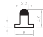
AC100_N0004 Joint gomme noir 5 x 4,9 mm 50 barres de 6 ml / paquet
