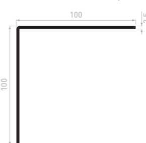
CE2520 Cornière 100X100X2,5 5 barres de 6 ml / paquet 250 barres de 6 ml / container
