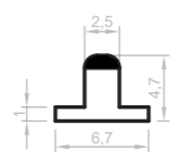
AC118_N0004 Joint gomme noir 6,7 x 4,7 mm 50 barres de 6 ml / paquet
