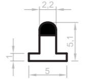
AC103_N0004 Joint gomme noir 5 x 5,1 mm 50 barres de 6 ml / paquet
