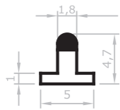
AC191_N0004 Joint gomme noir 5 x 4,7 mm 50 barres de 6 ml / paquet
