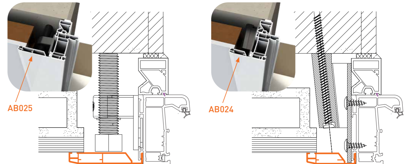
AB025 Moulure de 70 mm
