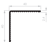
NEW CE2432C Cornière 40x40x2,4 crantée 10 barres de 6 ml / paquet 610 barres de 6 ml / container
