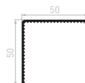
CE2535C Cornière 50X50X2,5 Crantée 10 barres de 6 ml / paquet 500 barres de 6 ml / container
