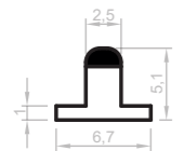
AC117_N0004 Joint gomme noir 6,7 x 5,1 mm 50 barres de 6 ml / paquet
