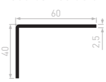
CE2530 Cornière 60X40X2,5 10 barres de 6 ml / paquet 500 barres de 6 ml / container
