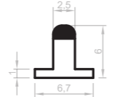
AC119_N0004 Joint gomme noir 6,7 x 6 mm 50 barres de 6 ml / paquet
