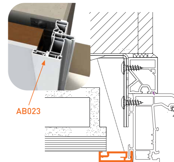
AB023 Moulure de 30 mm
