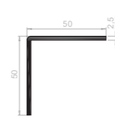
CE2535 Cornière 50X50X2,5 10 barres de 6 ml / paquet 500 barres de 6 ml / container
