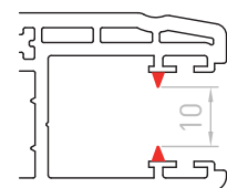
Montage du joint gomme sur coulisse PVC
