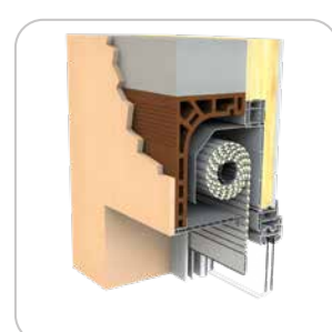
Pose en demi linteau maçonnerie
