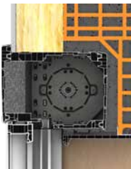
Pose en demi- linteau (R+1 accès par la trappe intérieure)
