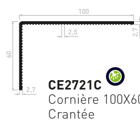
CE2720CS Cornière 100X100X2,7 Crantée sécable 5 barres de 6 ml / paquet 250 barres de 6 ml / container
