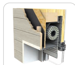
Pose sur maison ossature bois
