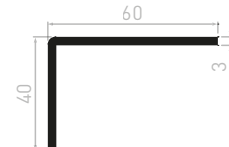
CE3030 Cornière 60X40X3 10 barres de 6 ml / paquet 400 barres de 6 ml / container
