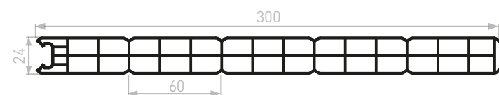
VB001 Panneau bi-cellulaire 300X24 pas de 60 3 barres de 6 ml / paquet 42 barres de 6 ml / container
