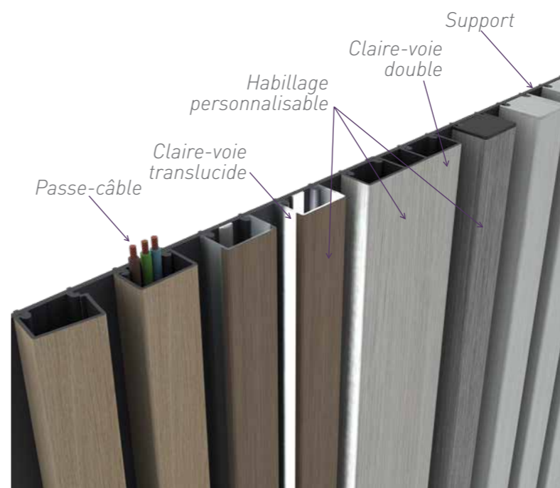
Le Block Art® comprend un profilé de base sur lequel se clipsent les différents profilés avec finition bois, pour créer un effet claire-voie traditionnel.
