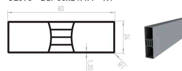
CL098 - Bar 80x24MM - R1
