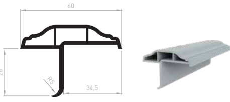
CL043 - Moulding - R5
