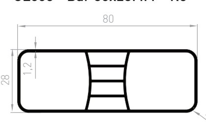
CL005 - Bar 80x28MM - R5
