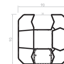
CL060 CL060U (CL060+CL054) Post, 3 slots 90 x 90
