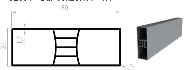
CL064 - Bar 80x28MM - R1
