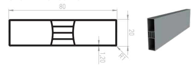
CL047 - Bar 80x20MM - R1
