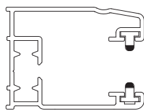
Plan de montage sur coulisse ALU
