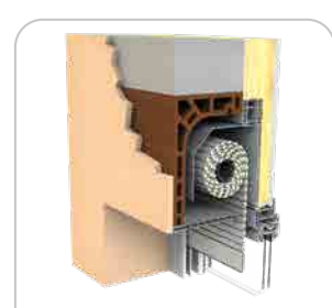
Pose en demi linteau maçonnerie
