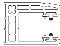
Plan de montage sur coulisse PVC
