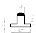
AC118_N0004 Joint gomme noir 6,7 x 4,7 mm
