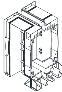
AC098 Embout Console Intermédiaire
