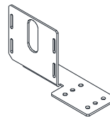
K344B6/B7 Equerre D120-160
