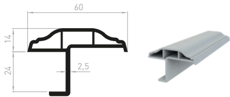
CL041 - Battement mouluré 24MM
