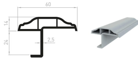
CL042 - Battement mouluré 24MM
