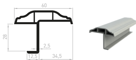
CL066 - Battement mouluré 28MM
