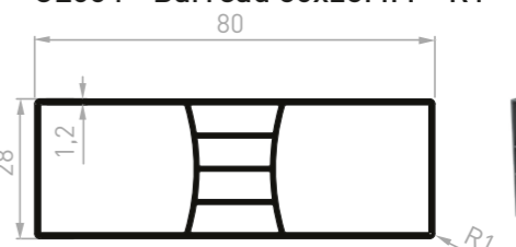
CL064 - Barreau 80x28MM - R1
