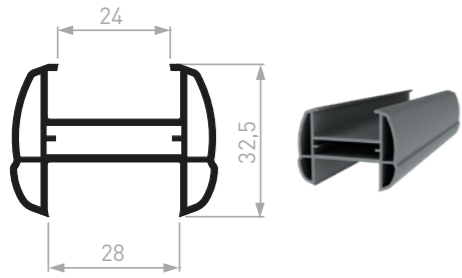
CL010 - Moulure à remplissage 24/28MM
