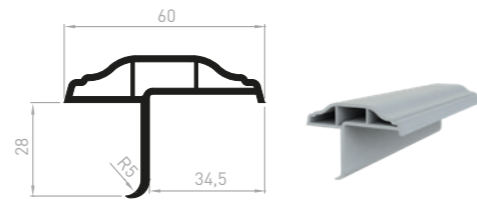
CL043 - Battement mouluré - R5
