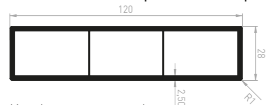
CL003 - 120x28 - R1 pour cintre uniquement
