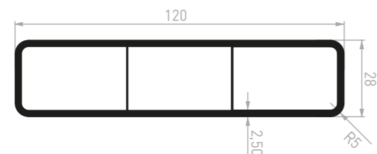
CL004 - Planche 120x28 - R5 pour cintre uniquement
