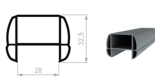
CL011 - Moulure à mortaiser 28MM
