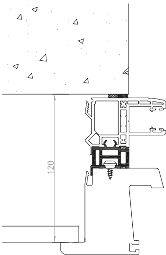
Montage en coulisse tapée
