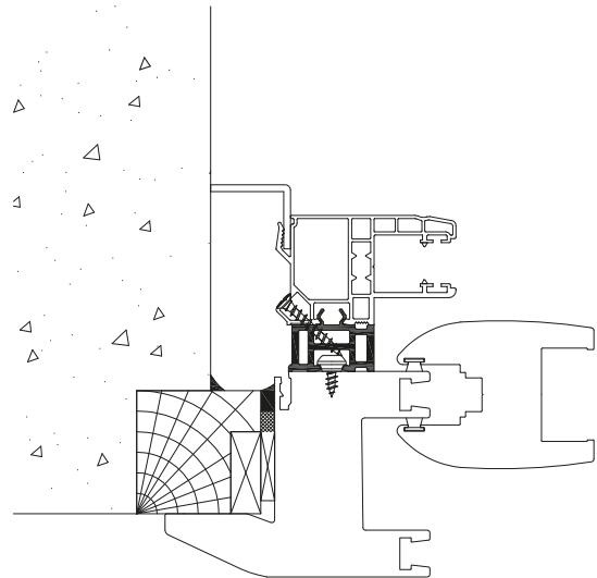
Montage en couissant
