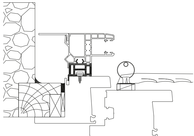
Montage en porte-serrure
